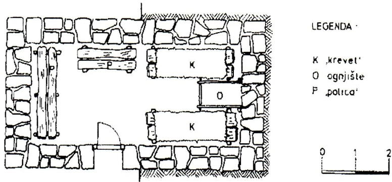
Crtež 1. Tlocrt KOLIBE, Police, planina Visočica
